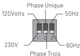
Figure 9: Interrupteurs DIP
