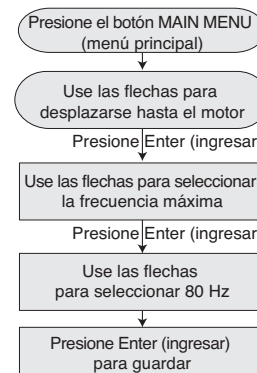
Figura 11 - Seleccione 80 Hz (solo para funcionamiento trifásico sumergible).
